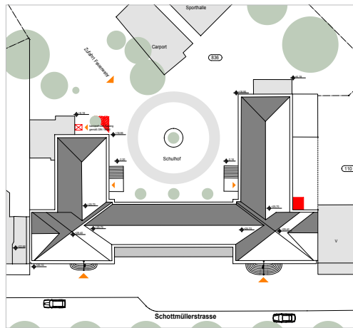
Lageplan
